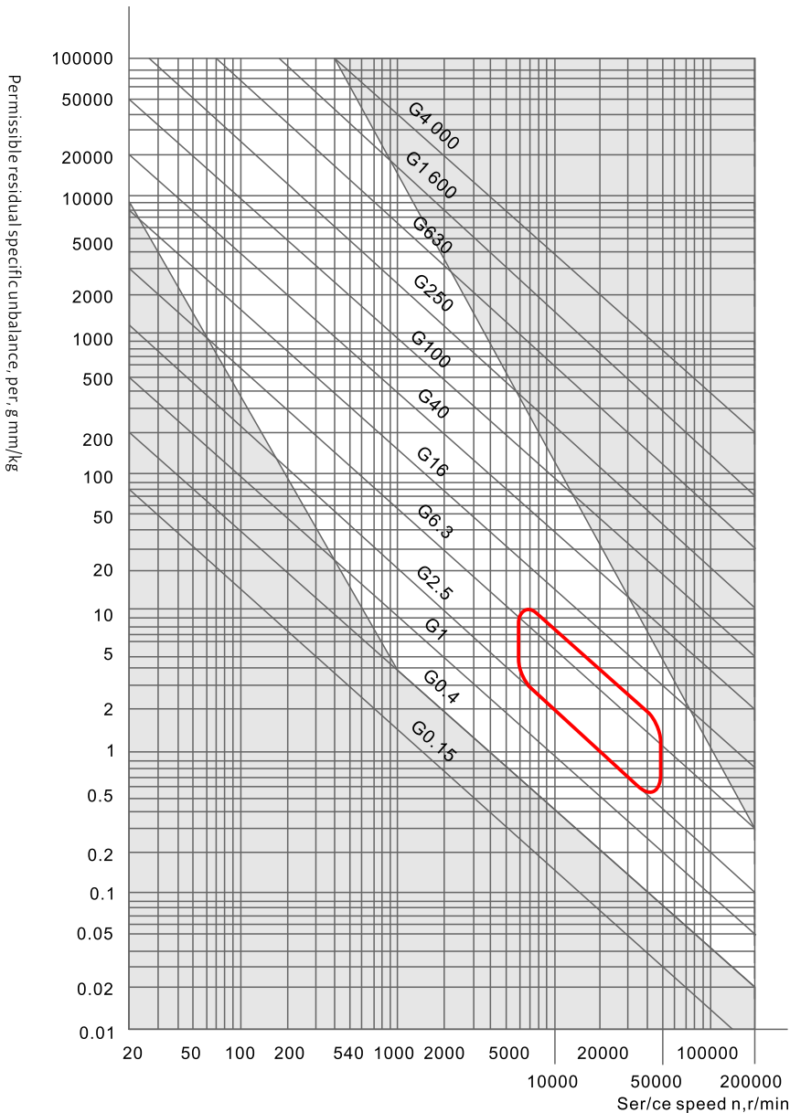
刀具动平衡推荐范围
