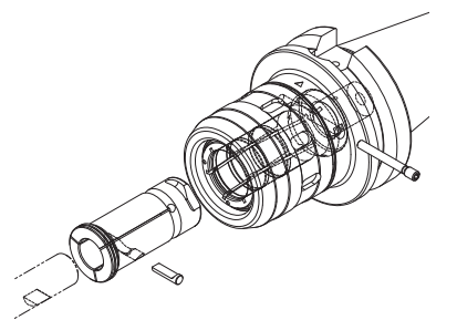
C-Lock强力夹头刀柄
